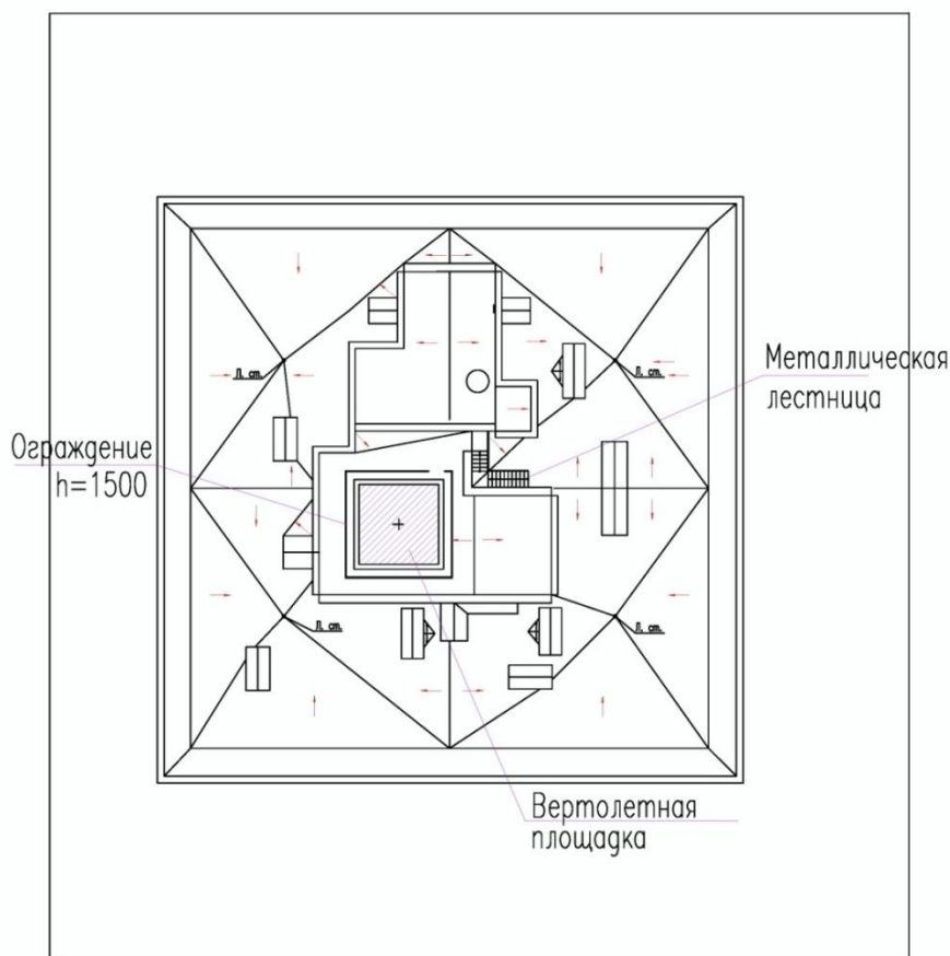
Рисунок 31 – План кровли с вертолетной площадкой
