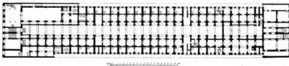
План подвала и первого этажа
