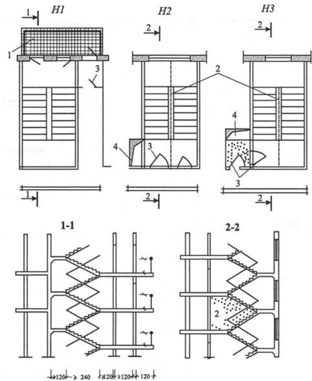
Рисунок 34 – Принципиальные схемы незадымляемых лестничных клеток
