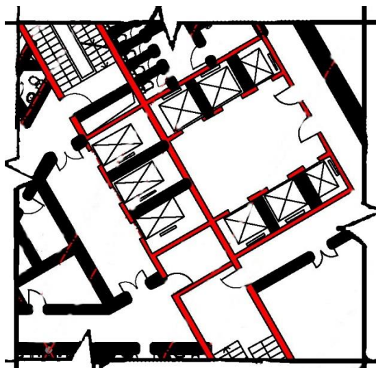
Рисунок 26 – Пример размещения лифтового холла
