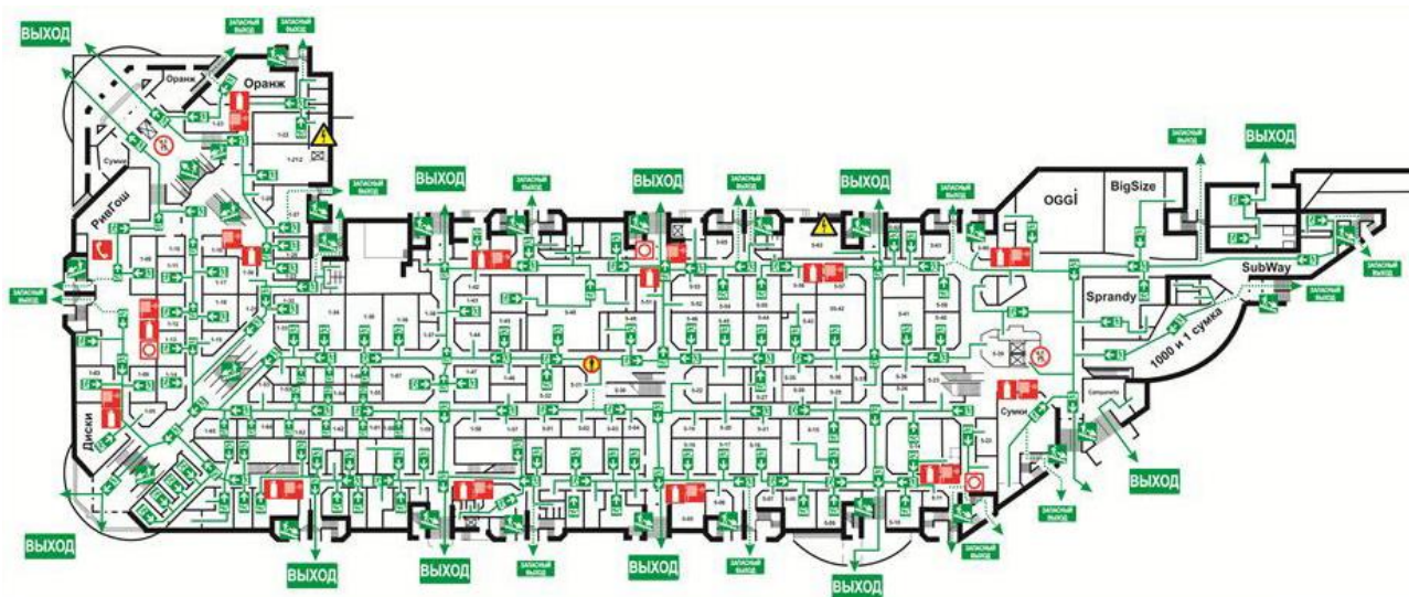
Рисунок 33 – Примерная схема эвакуации из многофункционального здания
