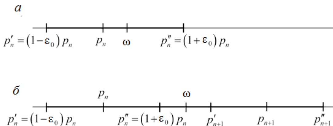
Рисунок 7.1 – Определение частот собственных колебаний
